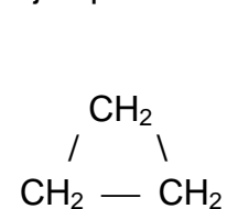
ciclopropano
