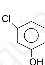
m-clorofenol
