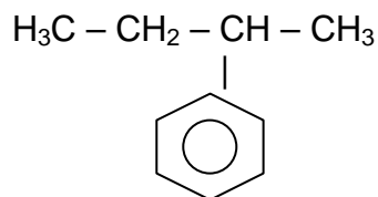
2-fenilbutano
