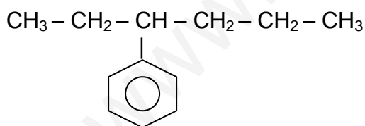
3 - fenilhexano
