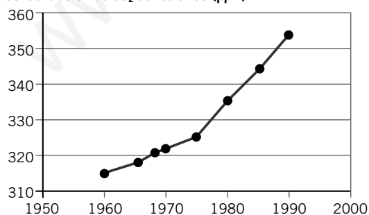
Concentración de \text{CO}_2 atmosférico (ppm)
