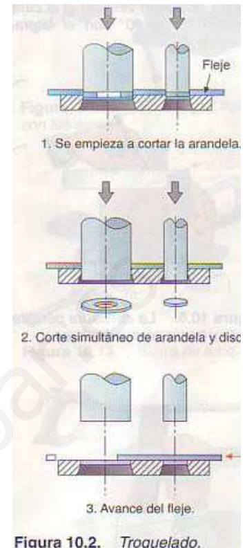
Figura 10.2. Troquelado.
