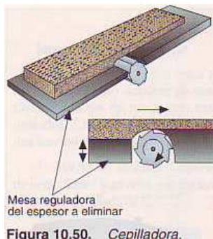
Figura 10.50. Cepilladora.
