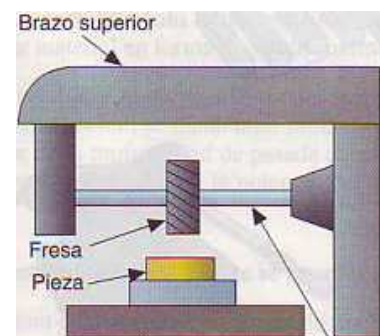
Figura 10.57. Vástago portafresas.
