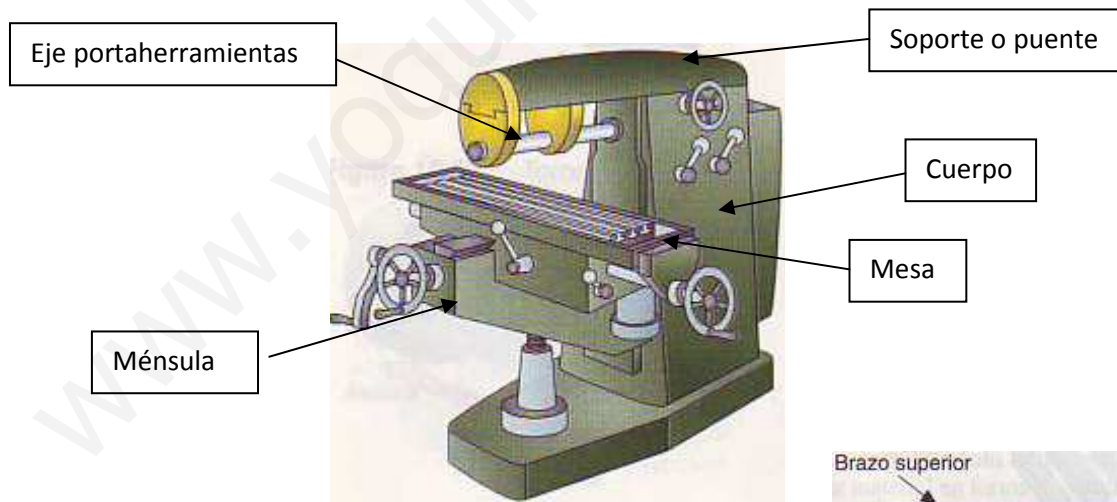
Figura 10.56. Fresadora.
