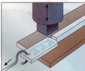
Figura 4.8(j). Acritud. Aumento de la dureza, fragilidad y resistencia en ciertos metales como consecuencia de la deformación en frío.
