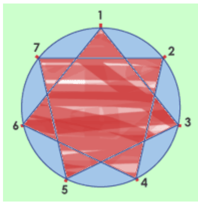
Polígono estrellado 7/2
