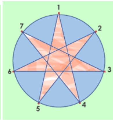
Polígono estrellado 7/3
