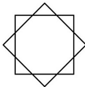
Estrella de 8/2
