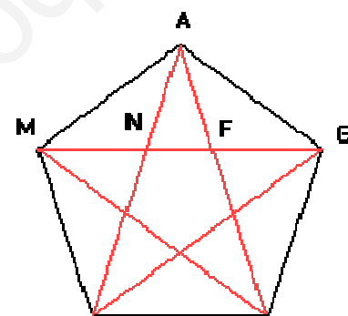
Polígono estrellado 5/2
