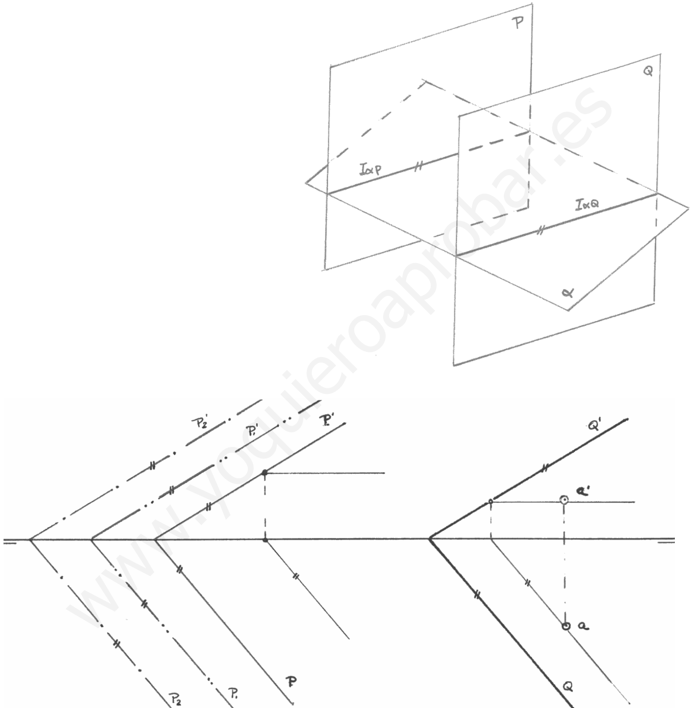
Fig. 50. Planos paralelos P, P_1, P_2, \dots Q .
