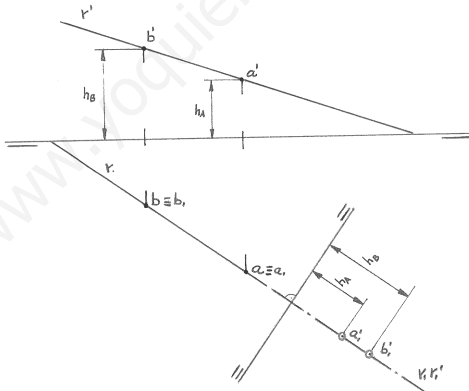
Fig. 71. Situar una recta cualquiera R como recta de perfil.
