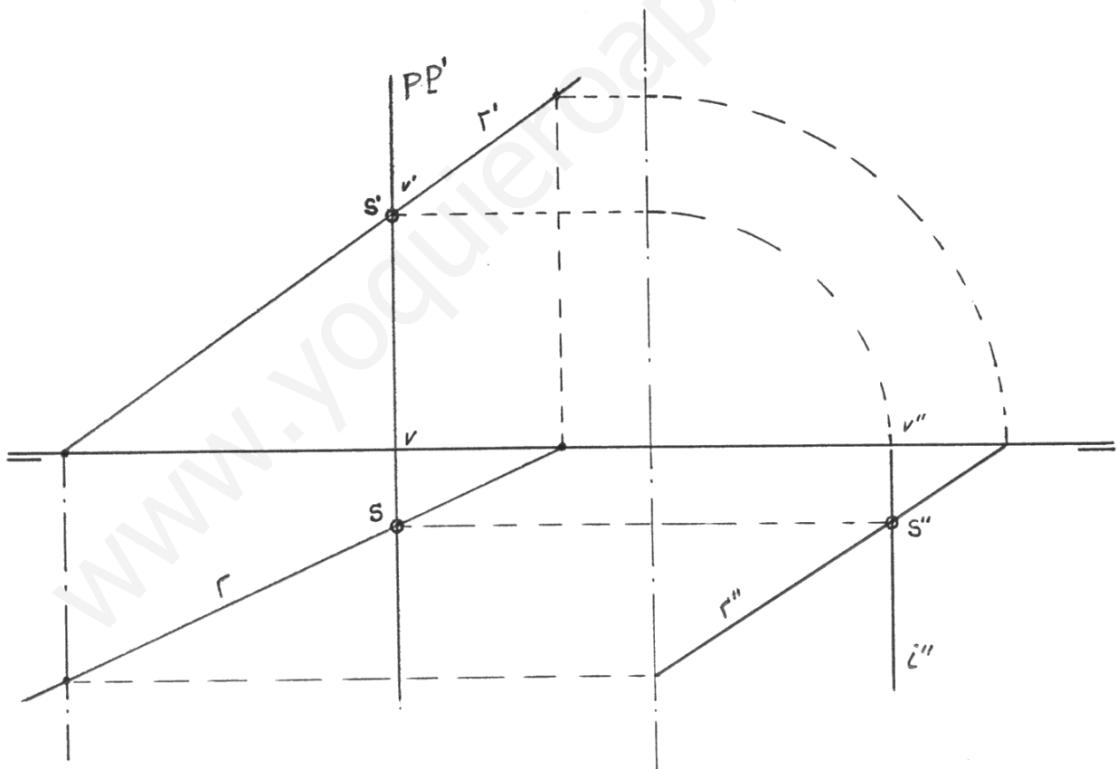
Intersección de una recta y un plano paralelo a la L.T.
