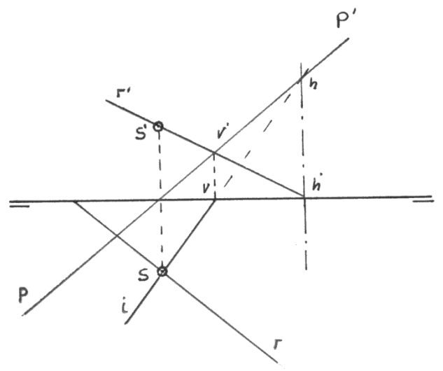
Intersección de una recta y un plano perpendicular al 2º bisector
