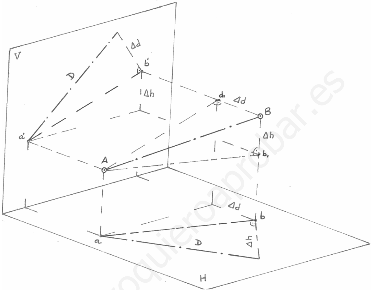
Fig. 57. Distancia entre dos puntos.
