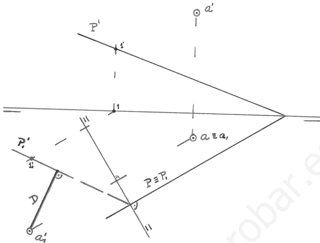
Fig. 78.1. Determinar la distancia de un punto A a un plano P .
