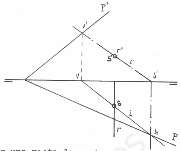
Intersección de un plano con una recta de punta.
