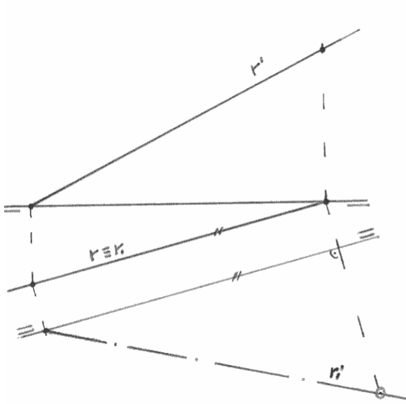
Fig. 69. Situar una recta cualquiera R como recta frontal.
