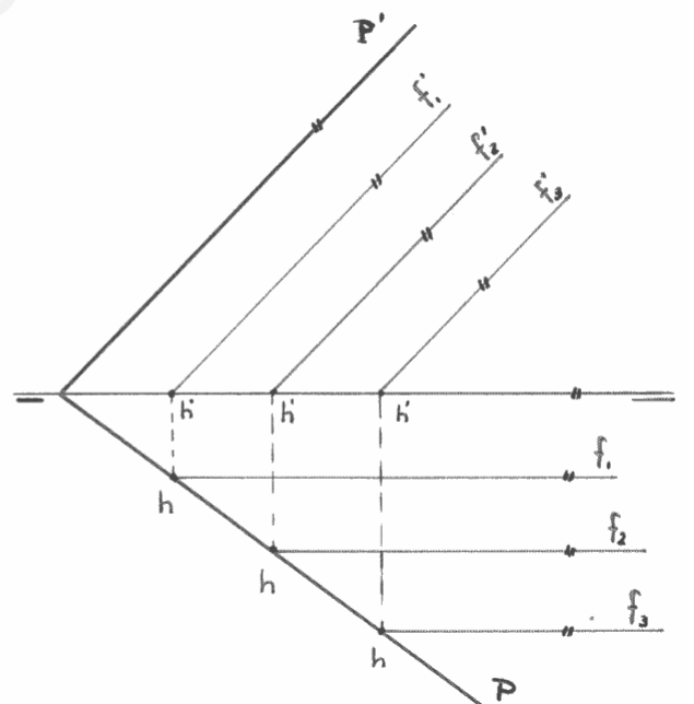
Fig. 28. Rectas horizontales y frontales del plano.
