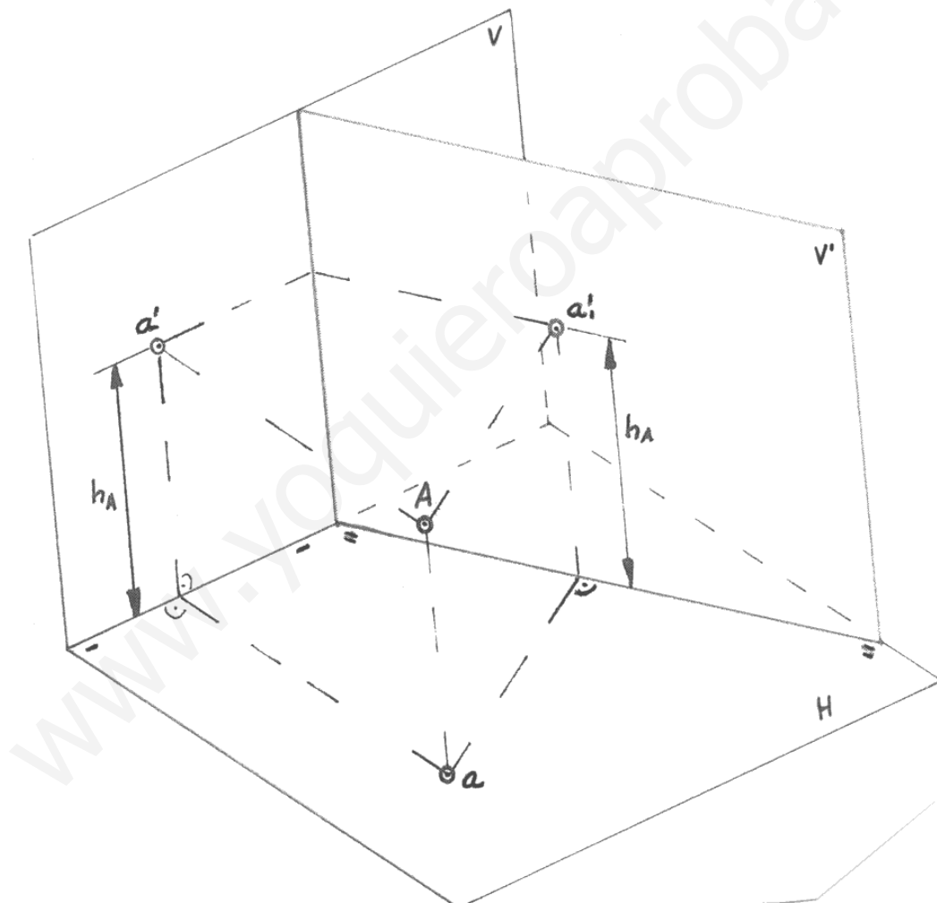
Fig. 64. Cambios de plano.
