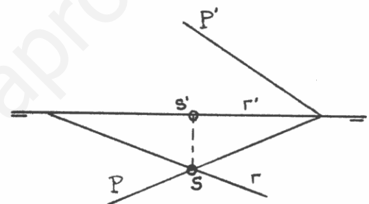
Intersección de un plano con una recta del plano Horizontal.
