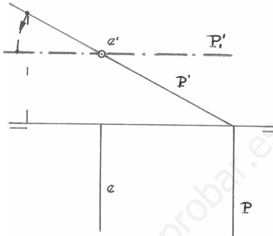
Fig. 91. Plano paralelo al horizontal.
