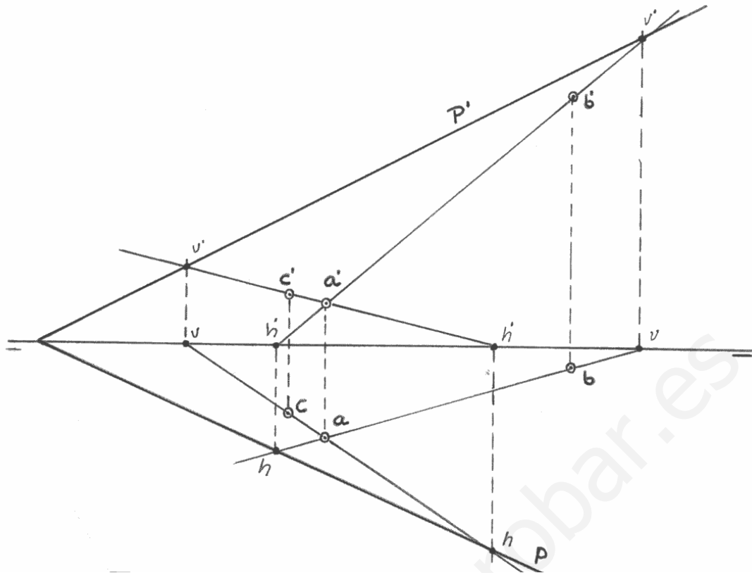
Fig. 22. Plano determinado por tres puntos ABC no alineados.
