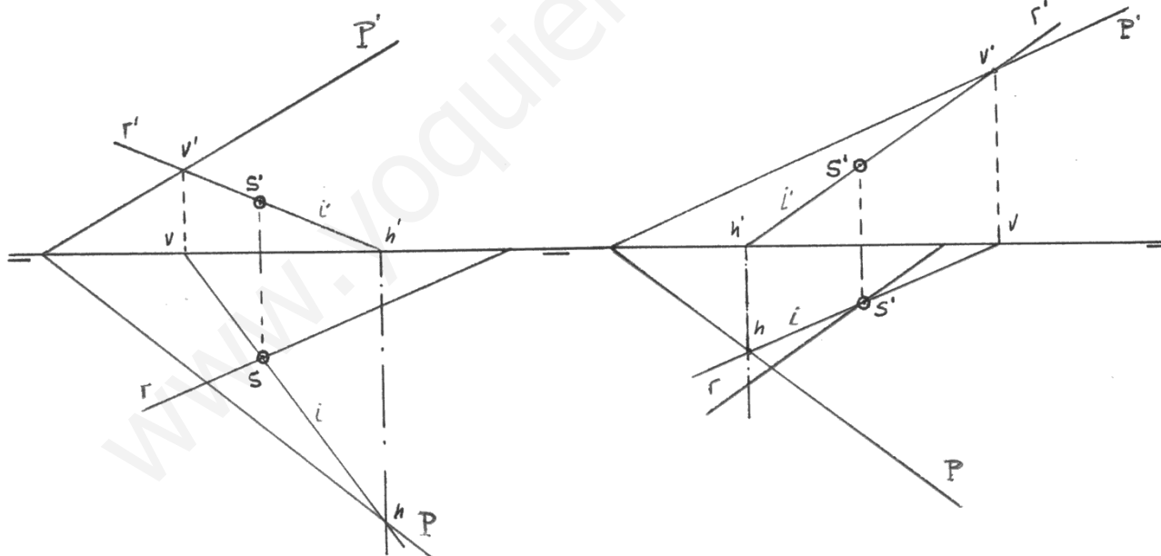
Intersección de un plano con una recta paralela al 1º bisector.
