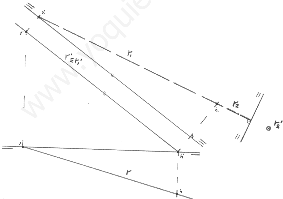
Fig. 73. Situar una recta cualquiera R como recta perpendicular al vertical.
