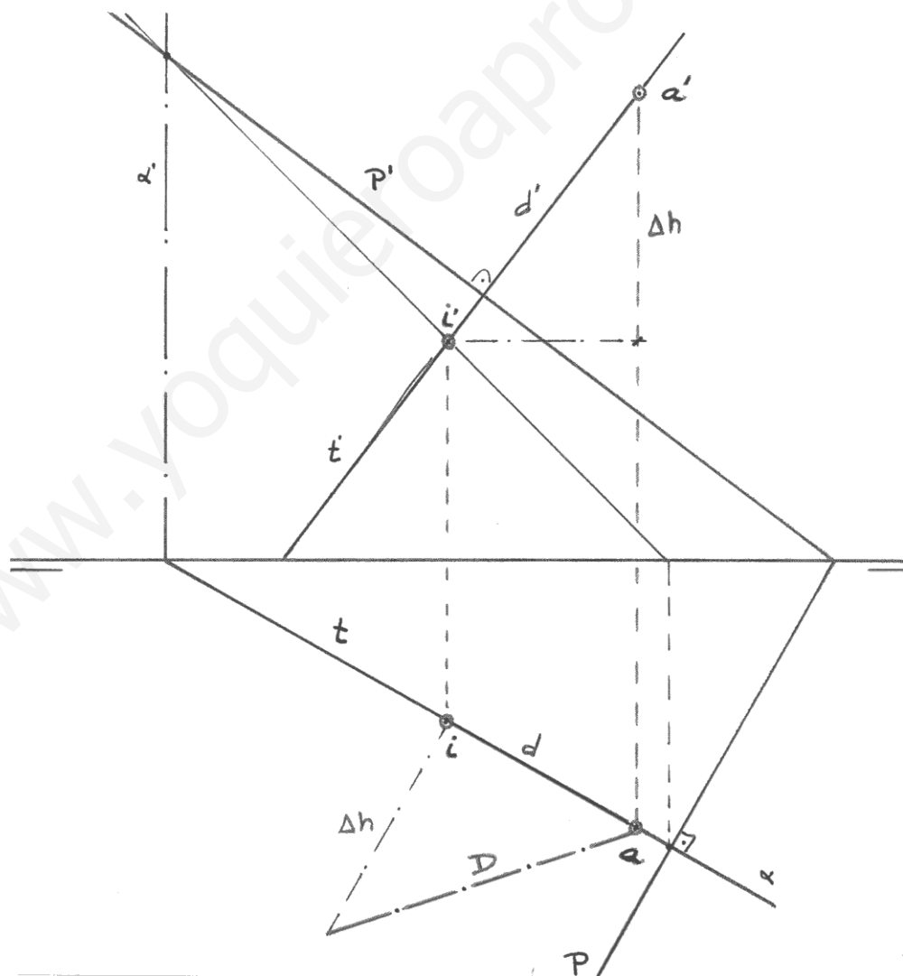
Fig. 59. Distancia de un punto A a un plano P.
