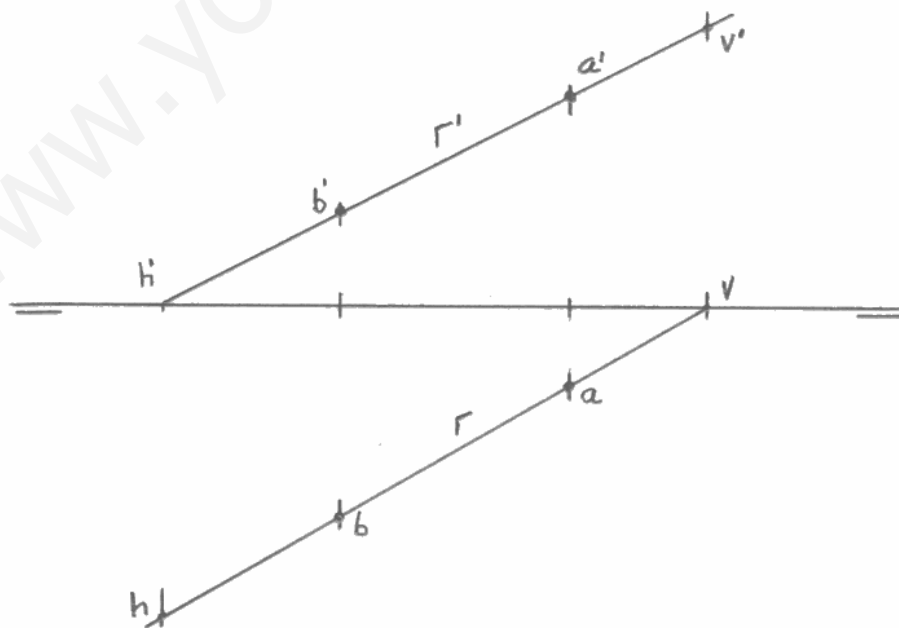
Fig. 5. Proyecciones de una recta.
