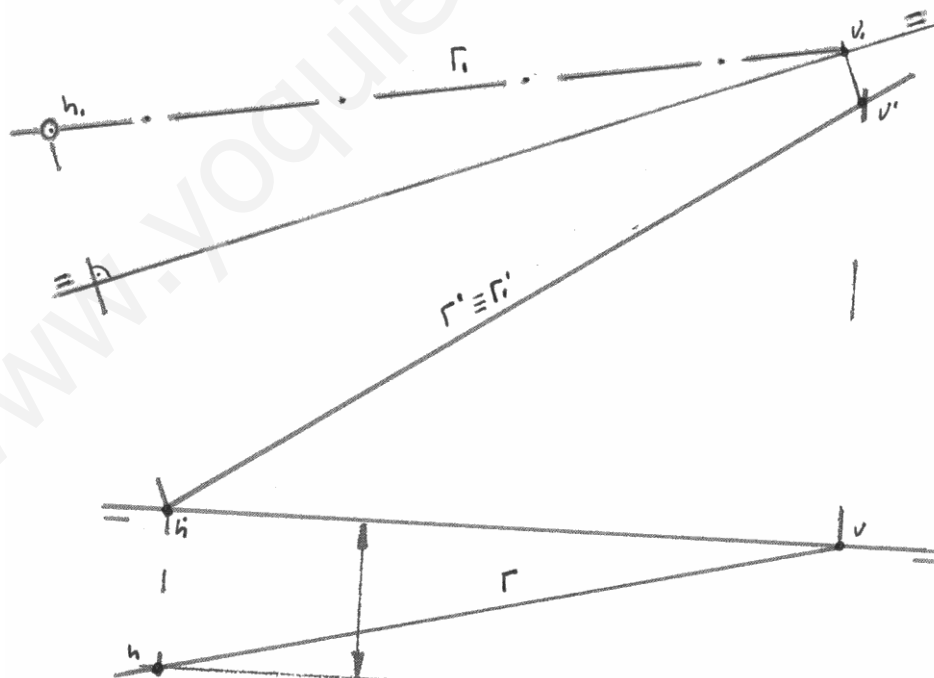
Fig. 68. Cambio del plano horizontal.
