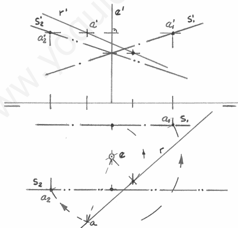
Fig. 84. Girar una recta R , alrededor de un eje E , hasta situarla como frontal.
