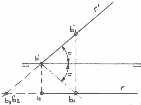
Fig. 10. Recta frontal.
