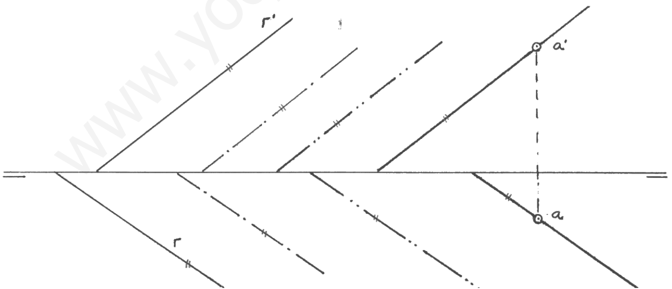
Fig. 45. Rectas paralelas.
