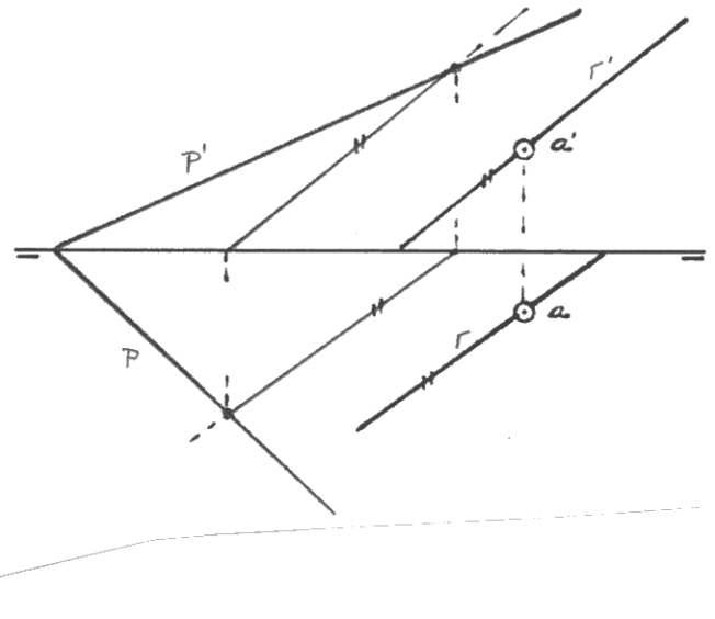
Fig. 47. Recta paralela a una recta de un plano.
