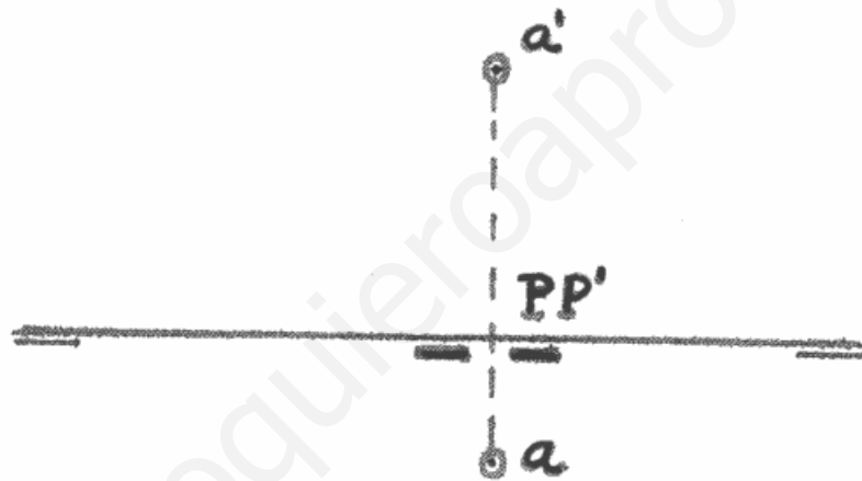
Fig. 37. Plano que pasa por la L.T.
