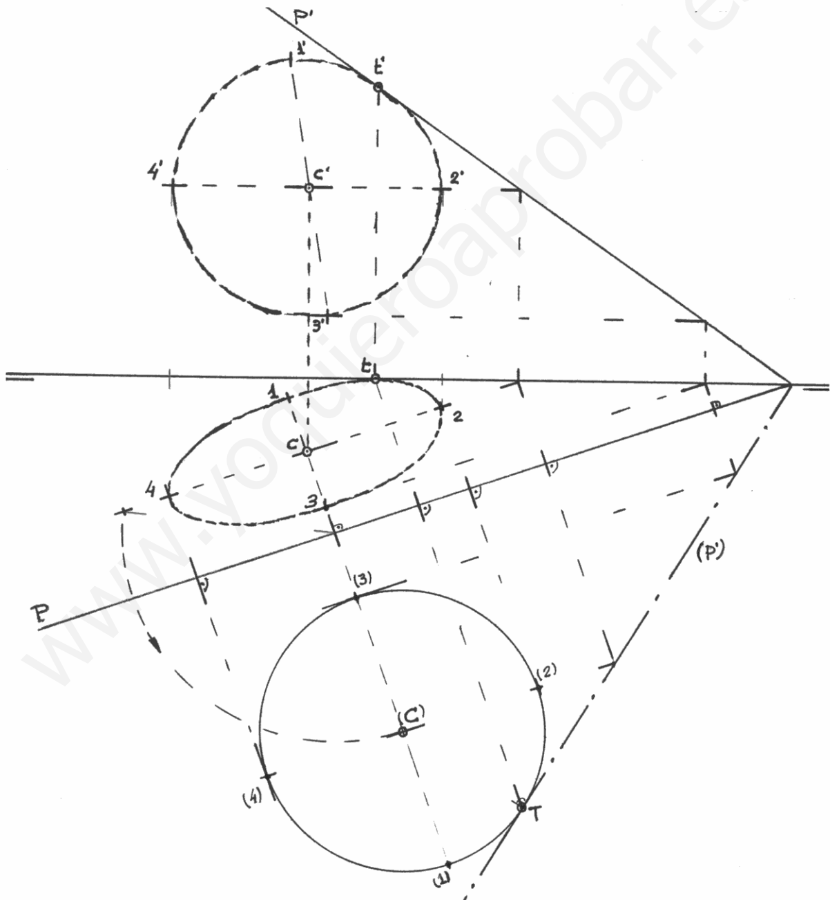
Fig. 99. Desabatimiento de una circunferencia.
