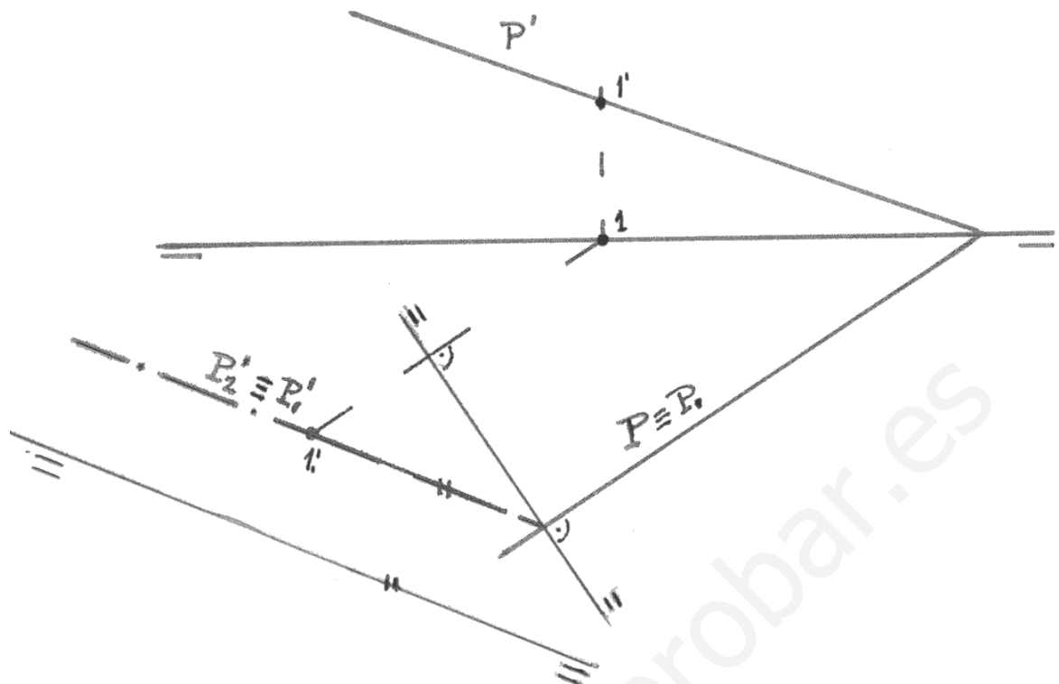
Fig. 77. Situar un plano cualquiera P como paralelo al horizontal.
