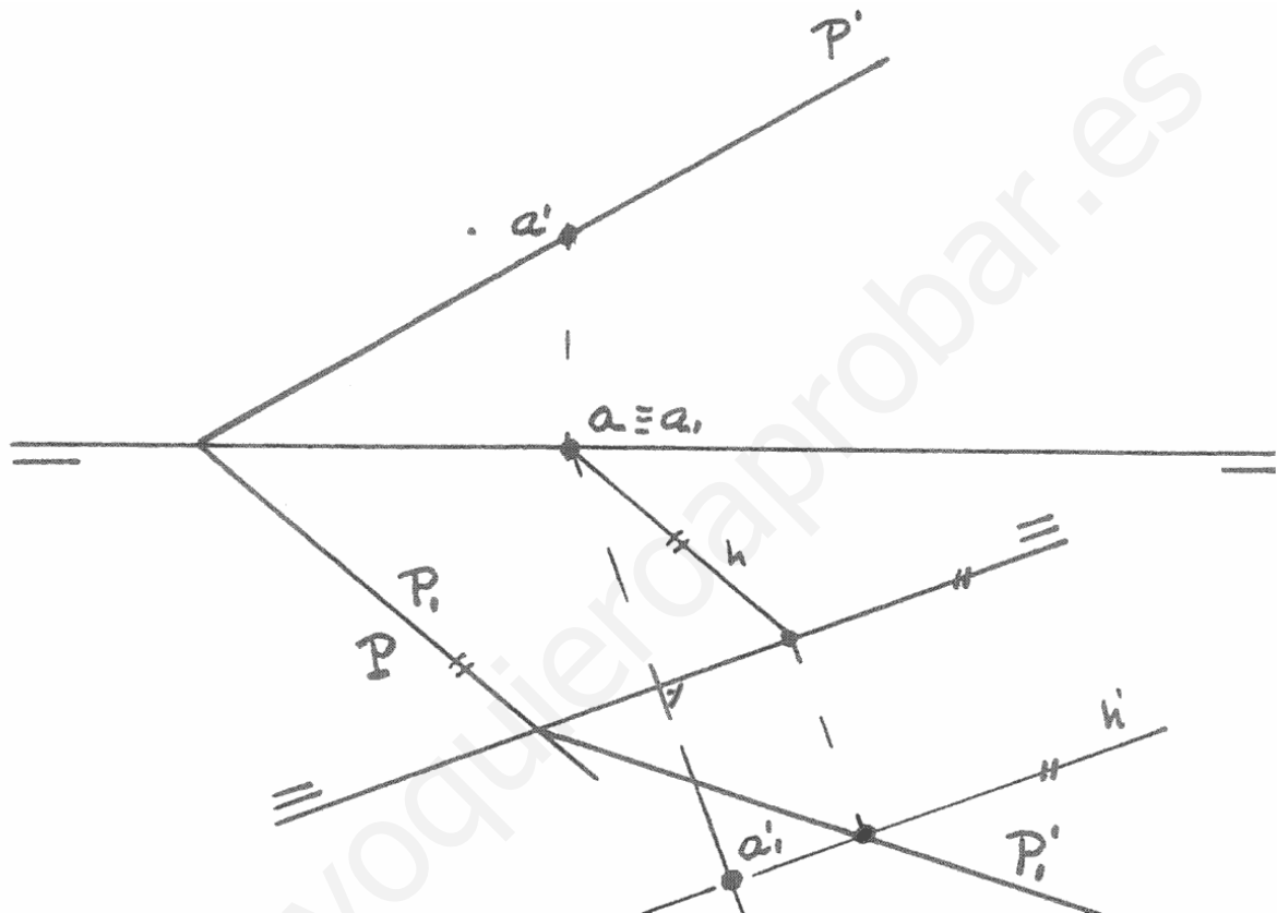
Fig. 74. Nuevas trazas del plano.
