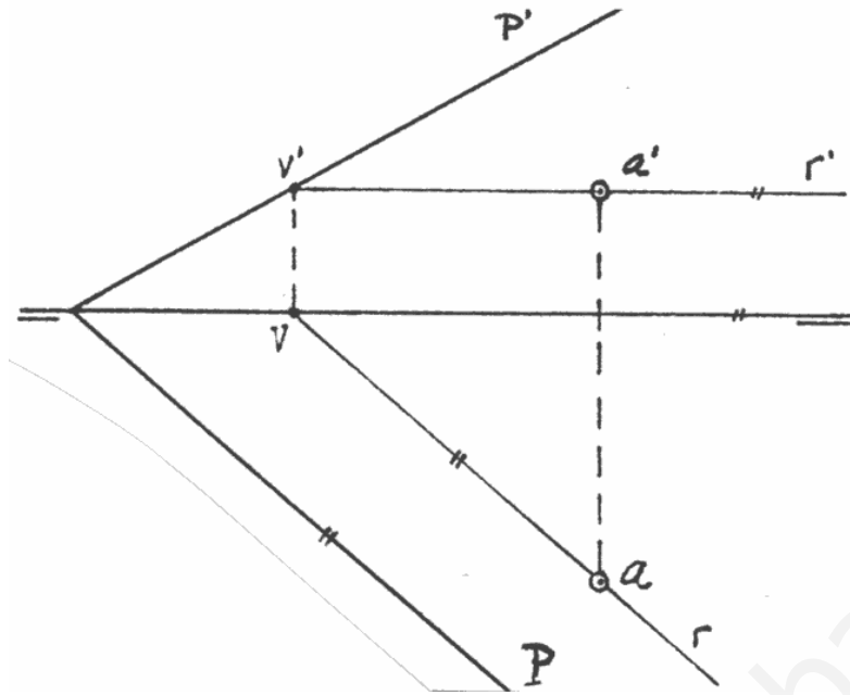
Fig. 26. Punto situado sobre un plano.
