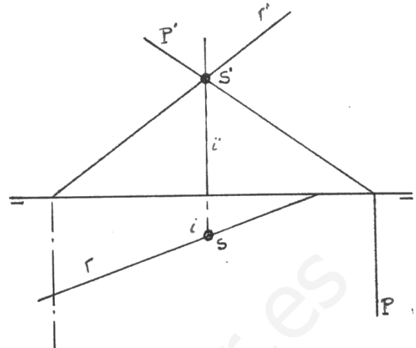
Intersección de una recta y un plano proyectante.
