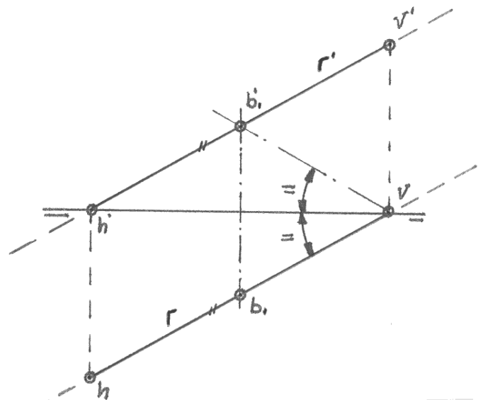
Fig. 19. Recta paralela al segundo bisector.
