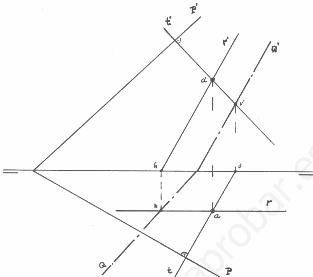
Fig. 55. Por una recta dada R trazar un plano Q perpendicular a un otro dado P.
