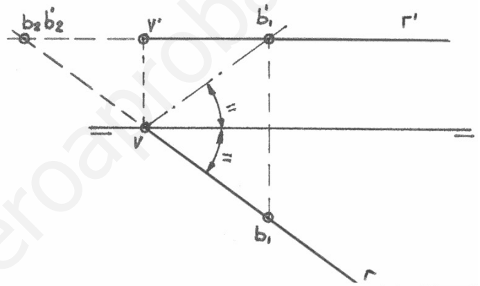
Fig. 11. Recta horizontal.
