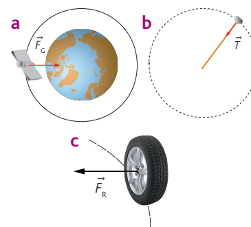
FIGURA 11 a Un satélite en órbita alrededor de la Tierra ( F_c = F_G ). b Una piedra atada a una cuerda que gira con movimiento circular uniforme ( F_c = T ). c Vista superior de un vehículo tomando una curva, y detalle de la fricción lateral entre el neumático y el asfalto ( F_c = F_f ). Si la fuerza de rozamiento es igual o superior a la fuerza centrípeta necesaria para tomar una curva a una determinada velocidad, el vehículo mantendrá la trayectoria esperada. En caso contrario, el automóvil se saldrá de la carretera, a no ser que el conductor reduzca la velocidad lo suficiente para que también disminuya la fuerza centrípeta exigida.
