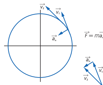
FIGURA 5 Un objeto se mueve con un MCU. El módulo de su velocidad se mantiene constante, pero la dirección varía continuamente. El vector \Delta \vec{v} representa la variación de velocidad de \vec{v}_1 a \vec{v}_2 ; su dirección es radial y su sentido hacia el centro de la circunferencia que describe (sentido centrípeto). La aceleración correspondiente \vec{a} y la fuerza resultante \vec{F} son también radiales y centrípetas.
