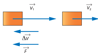
FIGURA 4 Un objeto con trayectoria rectilínea frena disminuyendo el módulo de su velocidad de v_1 a v_2 . El vector \vec{F} tiene la misma orientación que \Delta \vec{v} , y por tanto que \vec{a} (horizontal hacia la izquierda).
