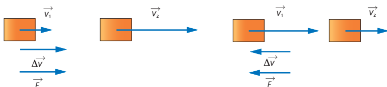
FIGURA 3 Un objeto con trayectoria rectilínea acelera aumentando el módulo de su velocidad de v_1 a v_2 . El vector \vec{F} tiene la misma orientación que \Delta \vec{v} , y por tanto que \vec{a} (dirección horizontal hacia la derecha).
