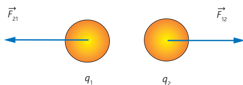
FIGURA 6 Representación de las dos fuerzas con que se repelen dos cargas de igual signo.
