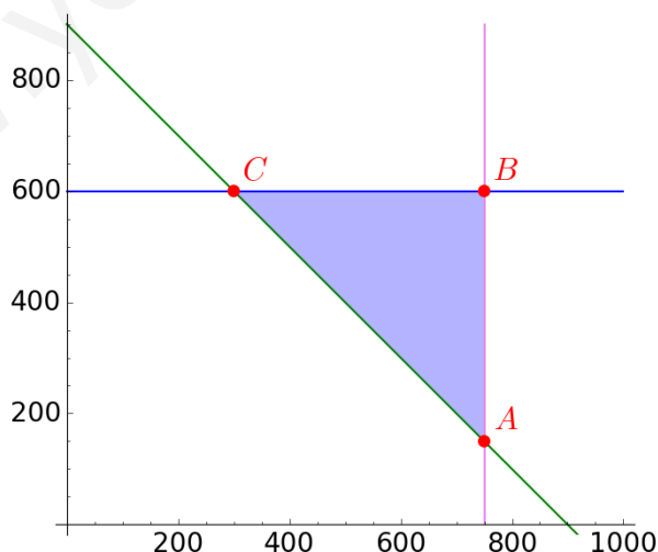
Figura 2: Región factible.
