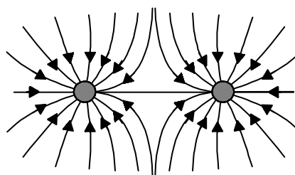
Líneas de campo gravitatorio generado por dos masas puntuales.
