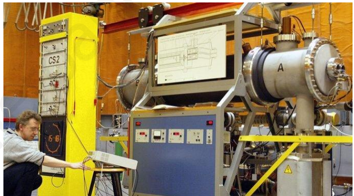
Reloj atómico de Cesio (NPL –CsF2)
