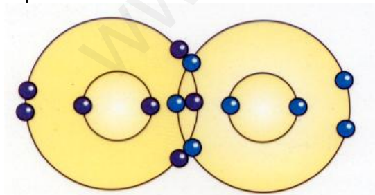
Ejercicios 21: Molécula de \text{N}_2 .
