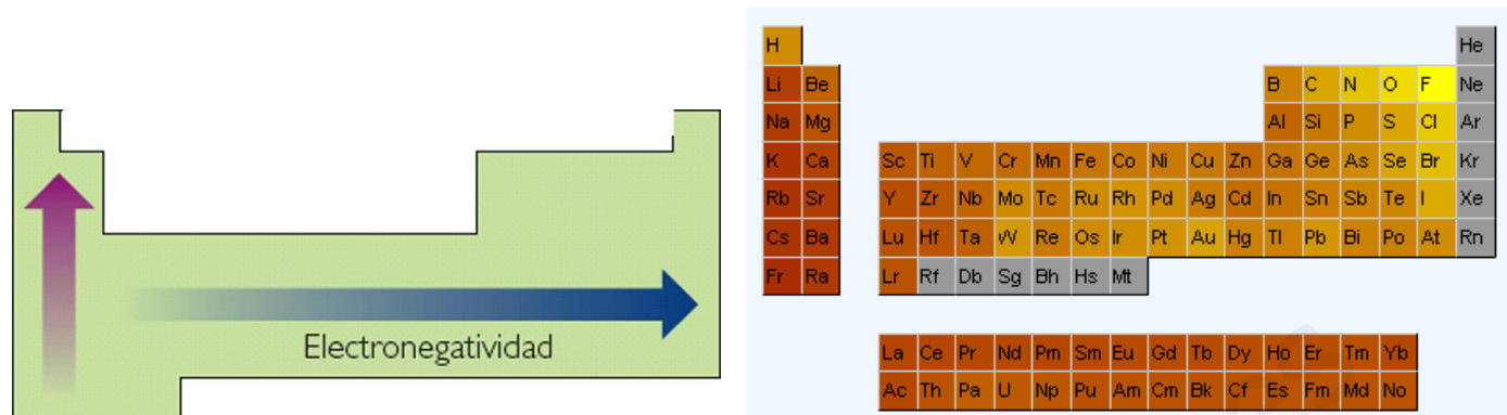
Aumento de la electronegatividad en la tabla periódica.
