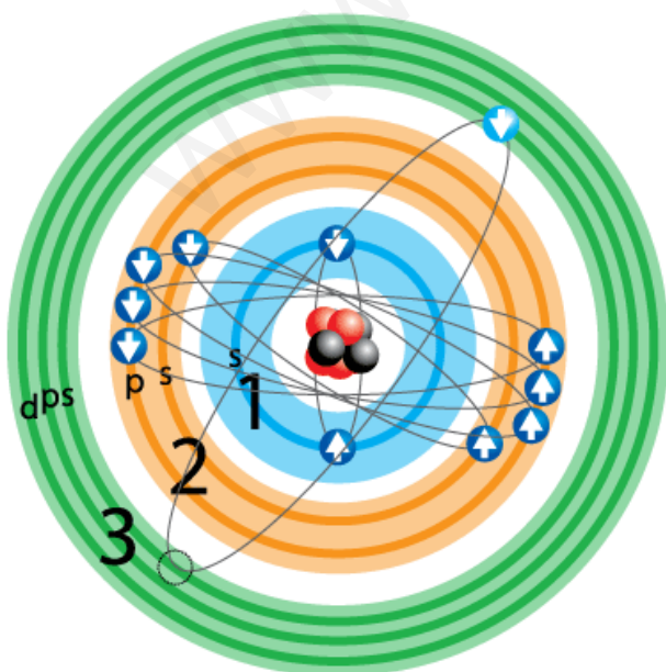
Sodio (Na)
