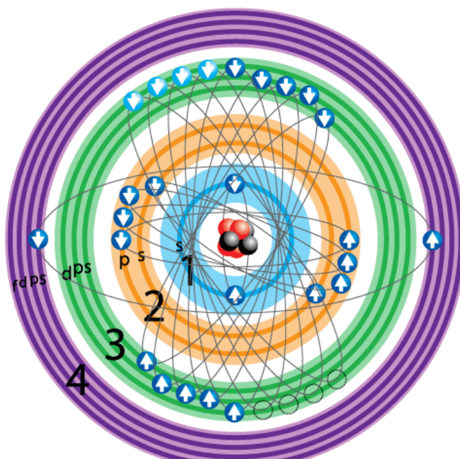
Hierro (Fe)
