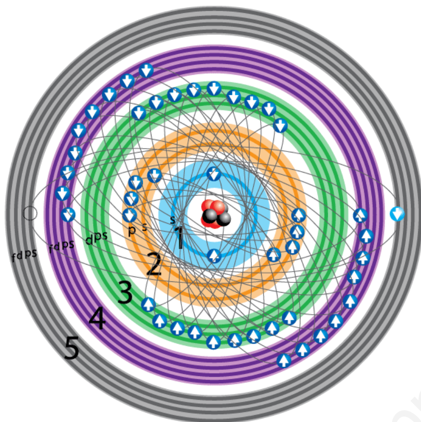
Plata (Ag)
